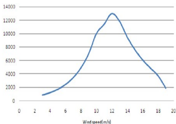
Teljesítménygörbe
